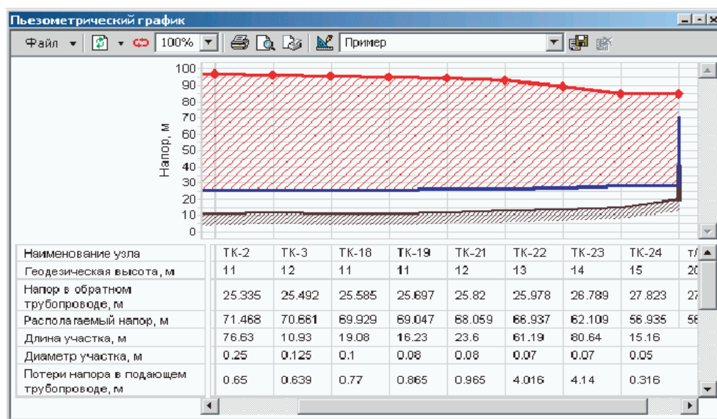
Рисунок 12.30 - Пьезометрический график
