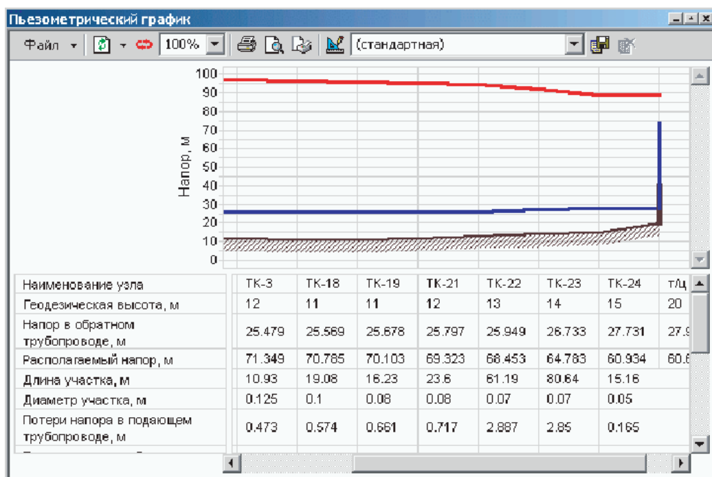
Рисунок 12.15 - Пьезометрический график
