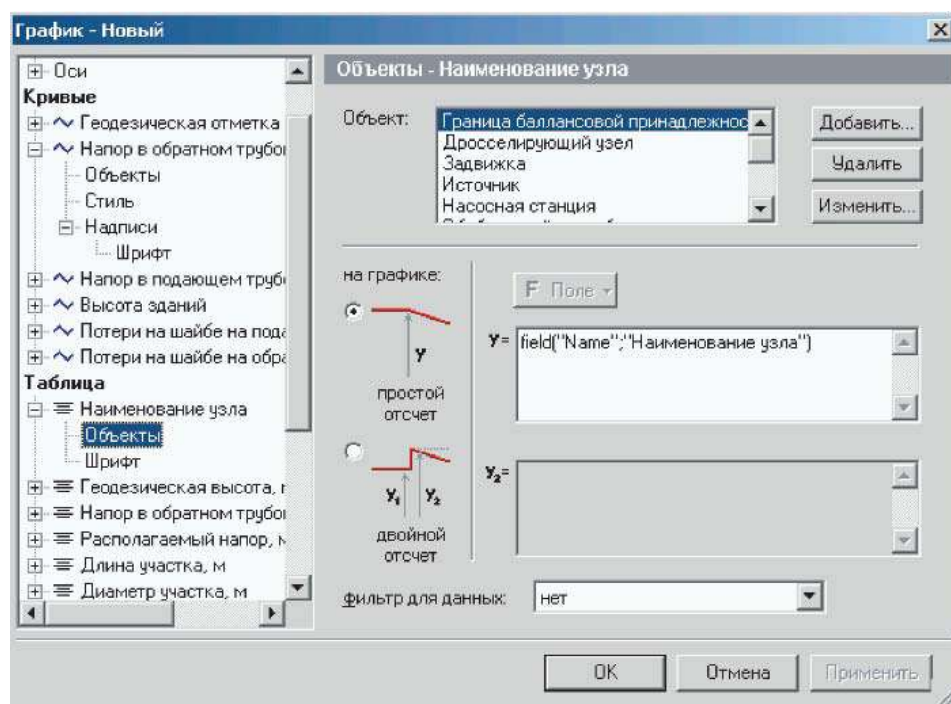
Рисунок 12.36 - Окно настройки графика Раздел Таблица
