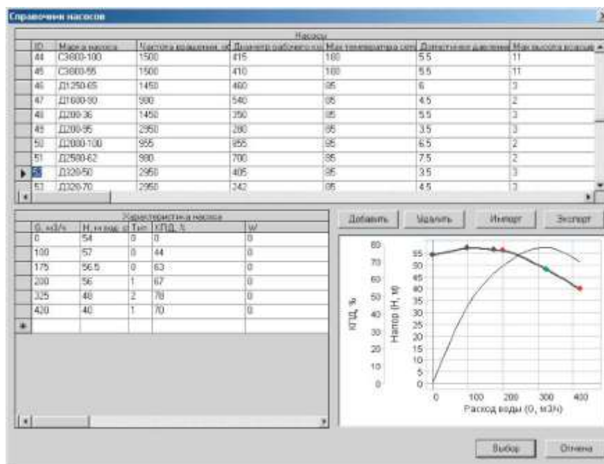
Рисунок 1.14 - Окно справочника по насосам
