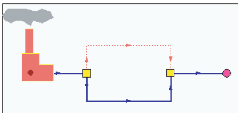
Рисунок 8.5 - Сеть с отключенным участком
