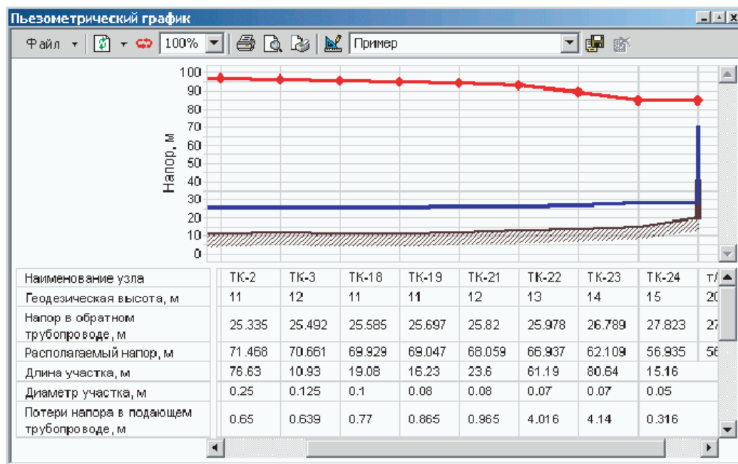
Рисунок 12.28 - Пьезометрический график
