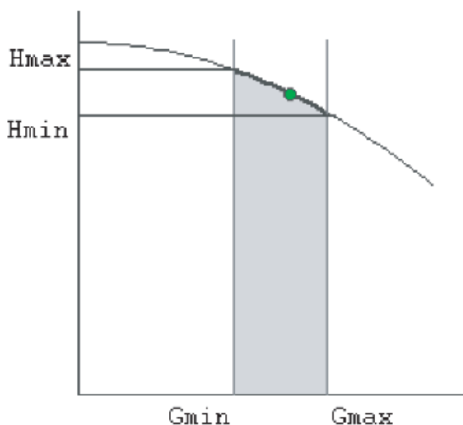
Рисунок 1.13 - Характеристика насоса
