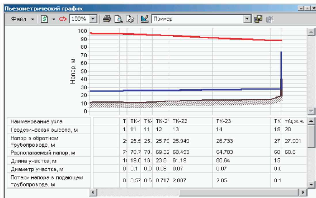
Рисунок 12.18 - Пьезометрический график
