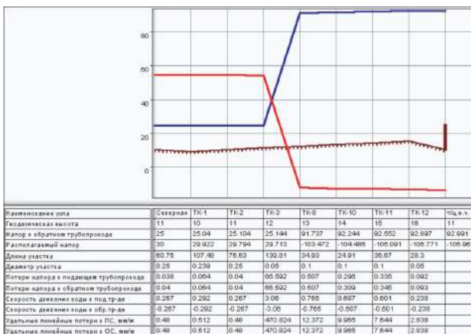
Рисунок 7.11 - Пьезометрический график
